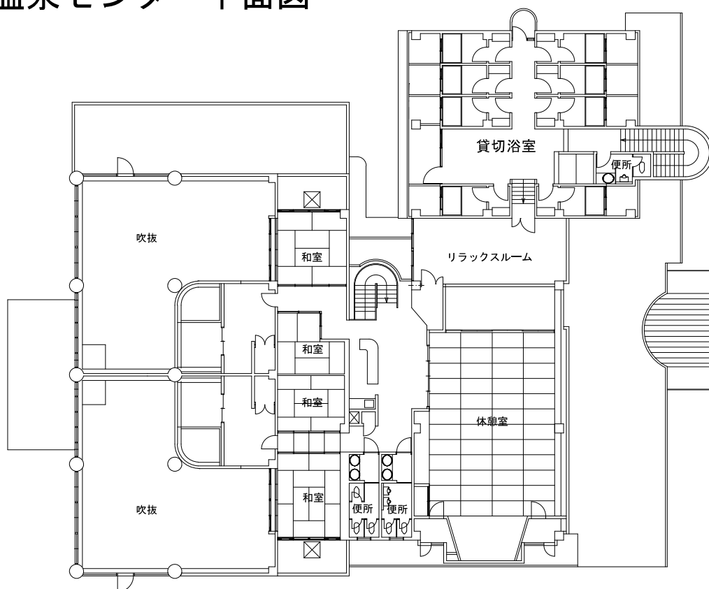
2階平面図
