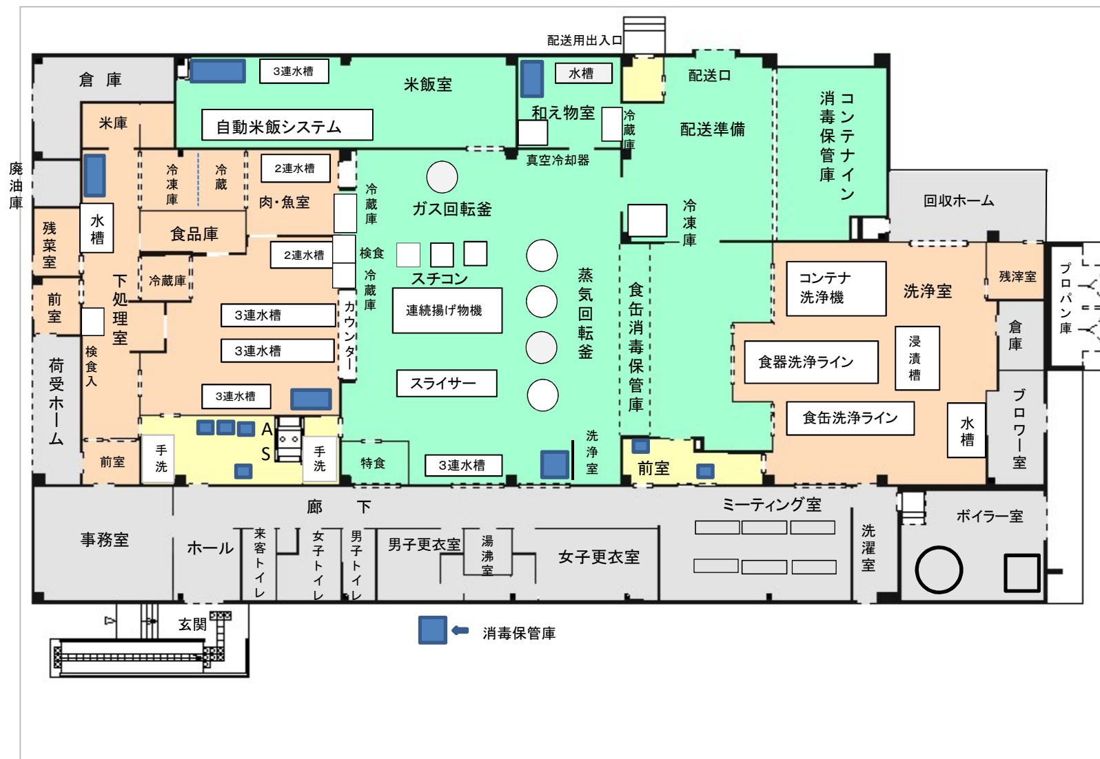
牛深学校給食センター 施設配置図
