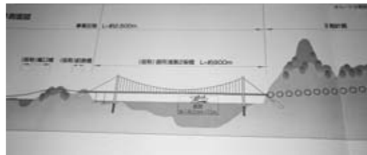
(仮称)御所浦第2架橋の側面図
