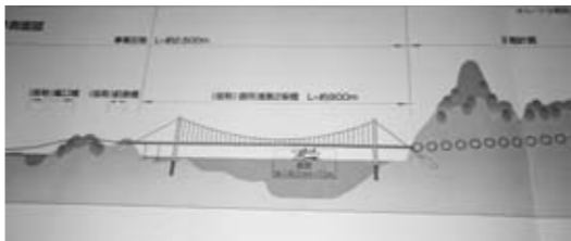
(仮称)御所浦第2架橋の側面図 出典：熊本県パンフレット
