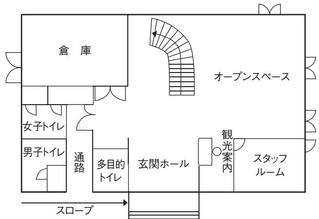
▲1階平面図
