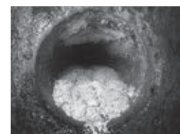
▲油の固まりで詰まった下水管
