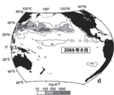
▲50年後の海洋表層のマイクロプラスチック重量濃度分布（環境白書より）
